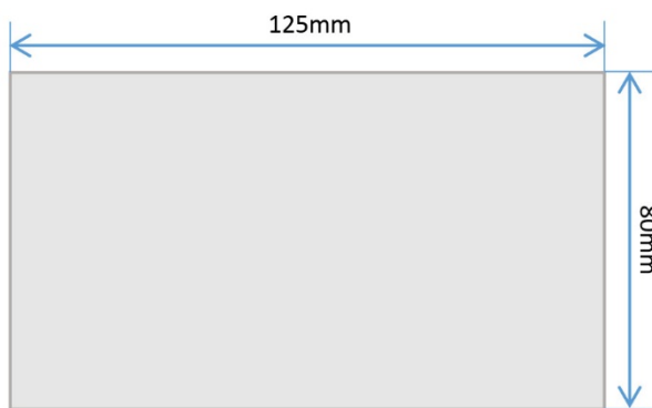
图1. BeyoGold™热封铝箔封板膜(FSF062)尺寸示意图。
